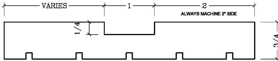
T-JAMB (1 3/4" DOOR)
