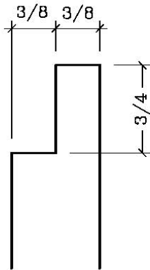
SIDE JAMB RABBET
